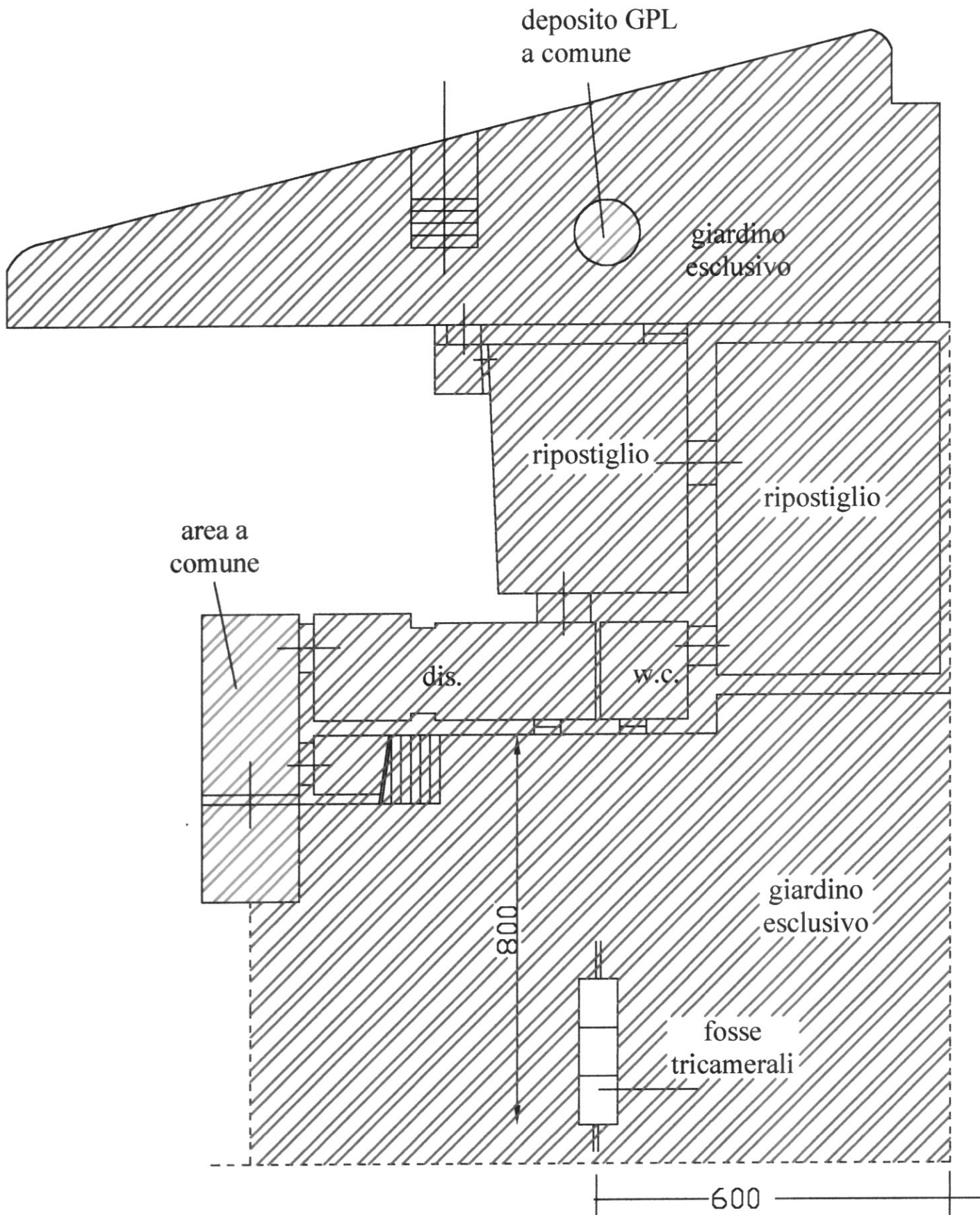
PIANTA PIANO TERRA FUORI SCALA
