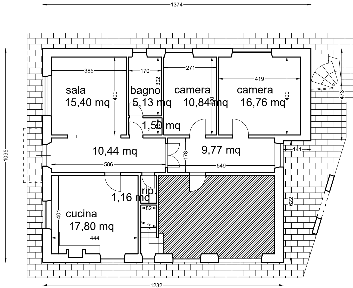
PIANTA PIANO TERRA 88,80 m 2 calpestabili
